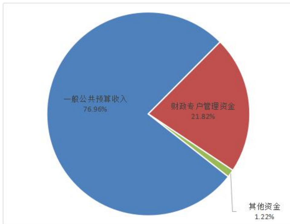
图1：收入预算图
