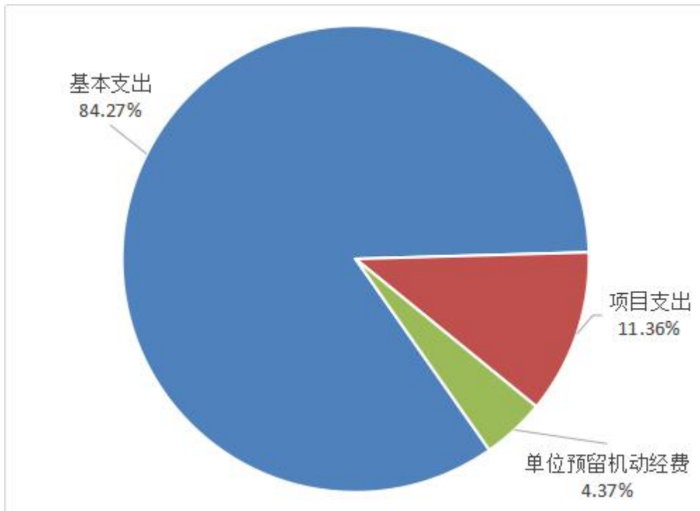
图2：支出预算图
